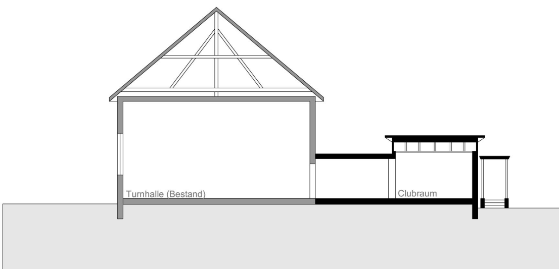
QERSCHNITT
